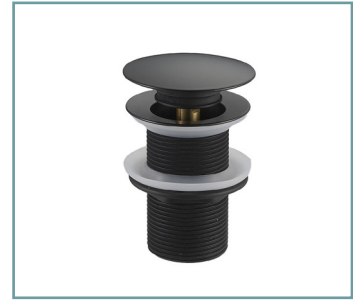
CLICK-CLACK leeresztő túlfolyó nélküli mosdóhoz drain for sink without overflow Szín/Color: Matt Black
